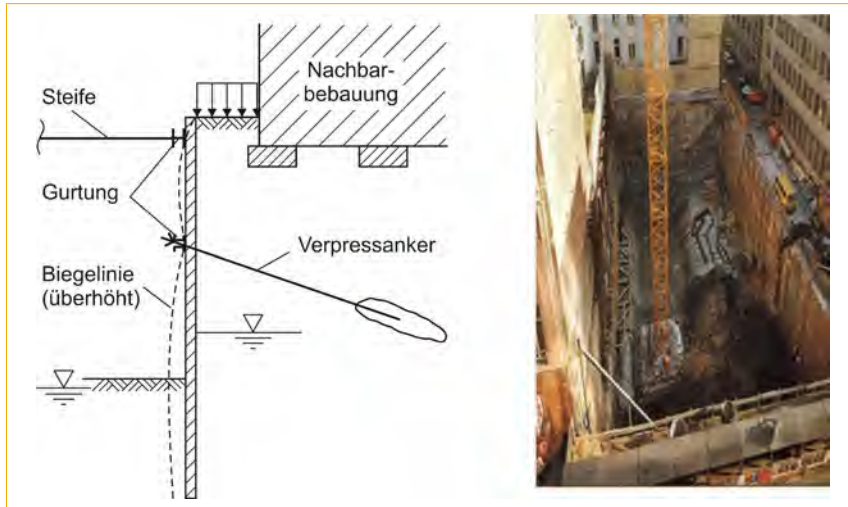
Abb. 02: Schemaskizze eines Baugrubenverbau (links) und Blick in eine tiefe Baugrube (rechts) [Quelle: Prof. Dr.-Ing. Martin Achmus]
