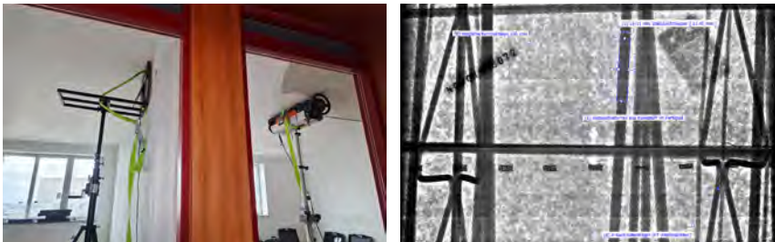
Abb. 05: Untersuchungsaufbau und Röntgenbild einer hochbelasteten Elementwand für das Anlegen von Kernbohrungen ohne Bewehrungstreffer und Fehlbohrungen: Erkennbar sind Bewehrungsstäbe, A-Böcke der Fertigteilshalen sowie Abstandhalter (Kunststoffräder). [Quelle: Dr.-Ing. Sebastian Schulze, bauray GmbH/hupfer ingenieure]
