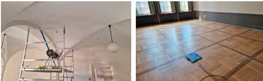
Abb. 06: Untersuchung einer denkmalgeschützten Eisenbetondecke per Radiographie: Messaufbau [Foto: Dr.-Ing. Sebastian Schulze, bauray GmbH]
